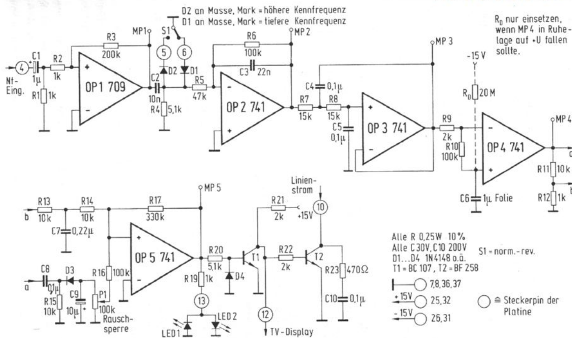
3.21 RTTY-Nf-Konverter DJ6 HP 025
